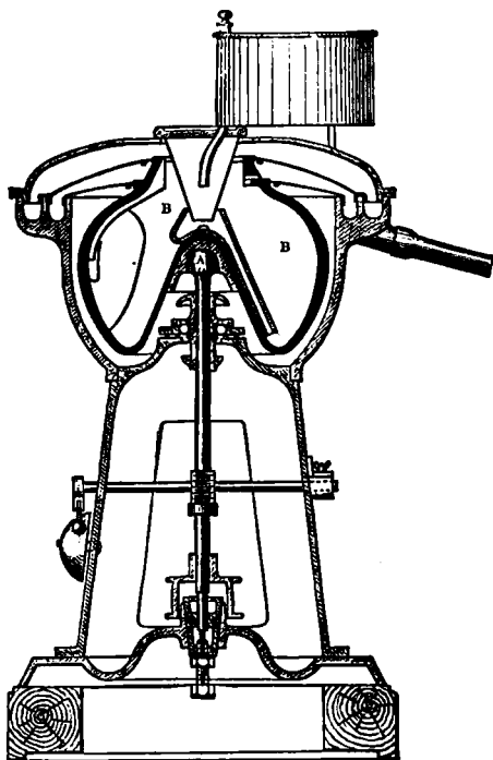
Fig. 17.— The Alexandra Separator.
